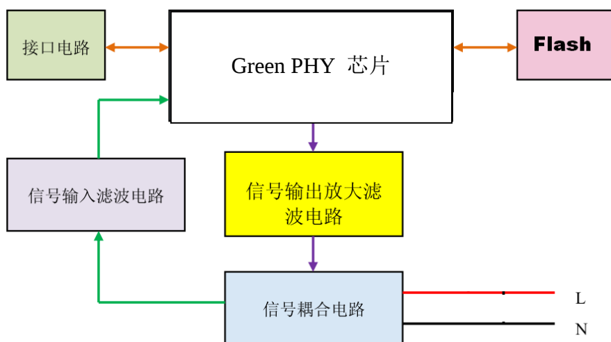
图 1 原理框图
