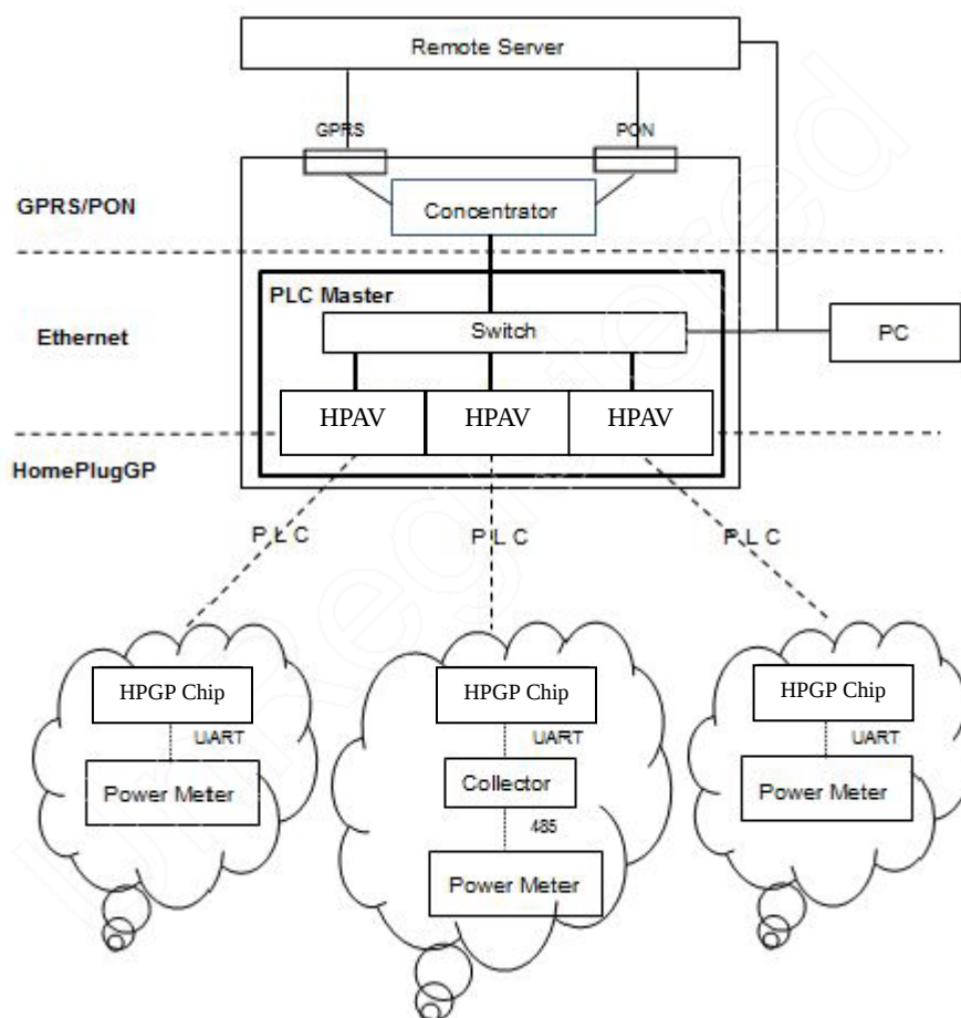
图2 宽带载波通信网络架构
