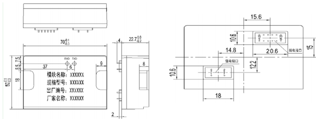
图 5 尺寸
