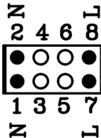
图 4 强电接口示意图
